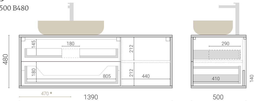
WPR 318 Д1210 Ш500 В480
