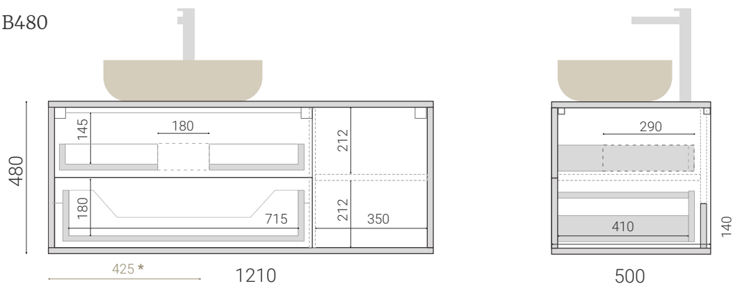
WPR 102 Д1300 Ш500 В480
