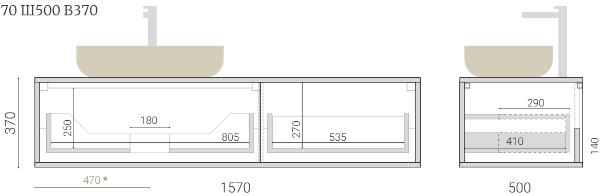
WPR 46 Д940 Ш500 В480
