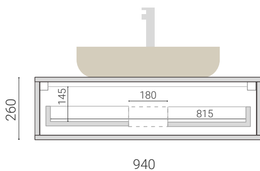
WPR 37 Д940 Ш500 В260
