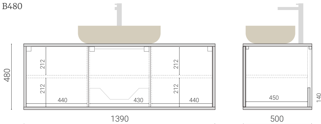
WPR 215 Д1480 Ш500 В480
