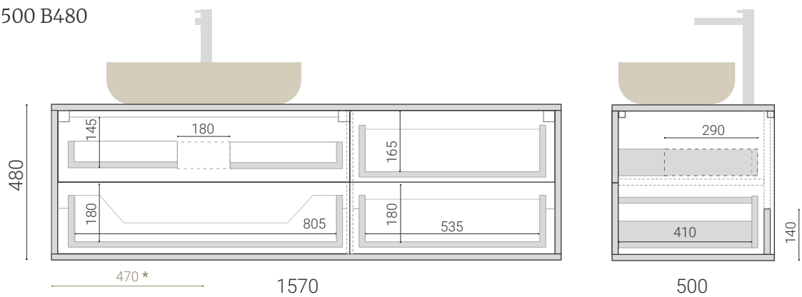
WPR 165 Д1660 Ш500 В590
