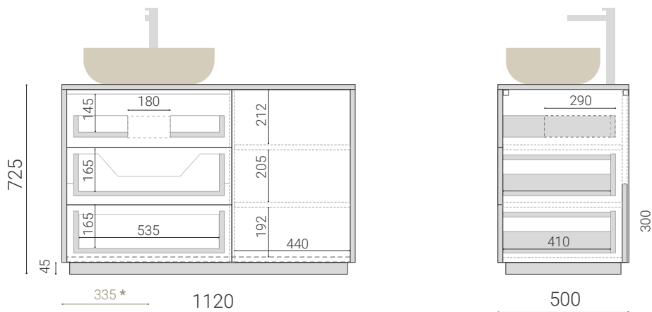
WPR 315 Д1120 Ш500 В725
