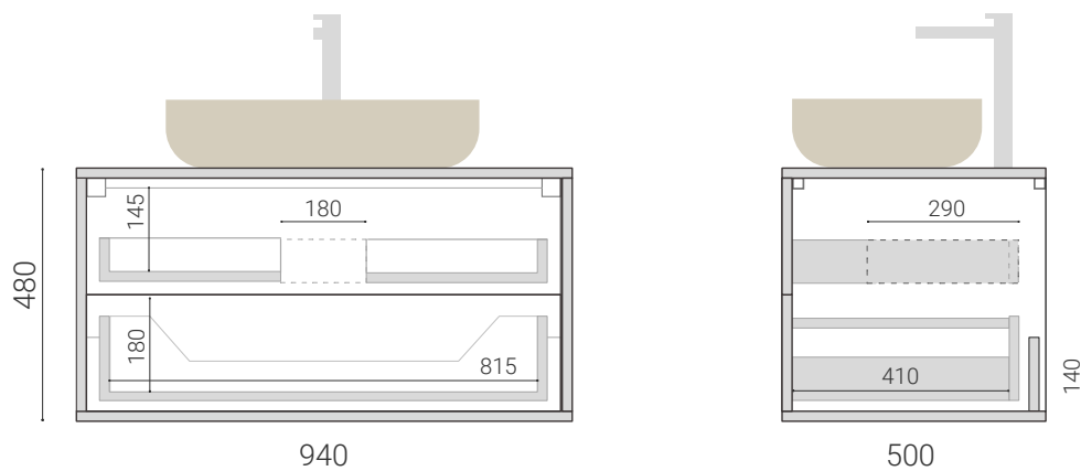
WPR 40 Д940 Ш500 В480
