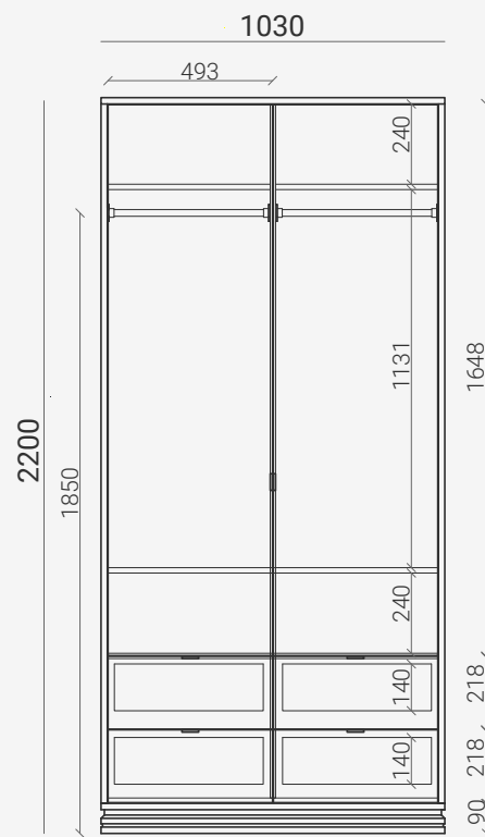
TLD212 Д1030 Ш600 В2200
