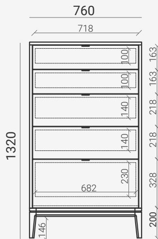
TL024 Д760 Ш450 В1320
