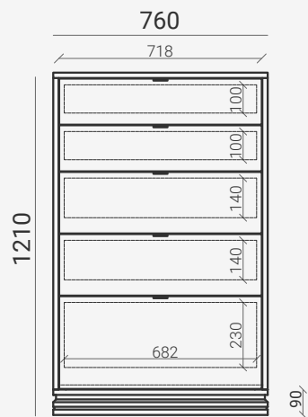
TLD024 Д760 Ш450 В1210
