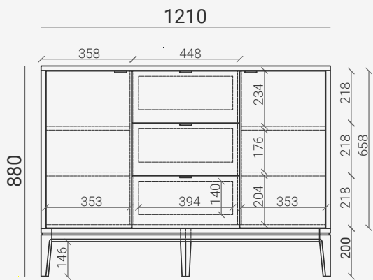
TL039 Д1210 Ш400 В880
