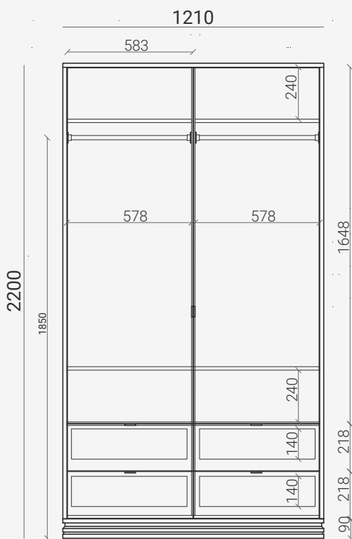
TLD217 Д1210 Ш600 В2200
