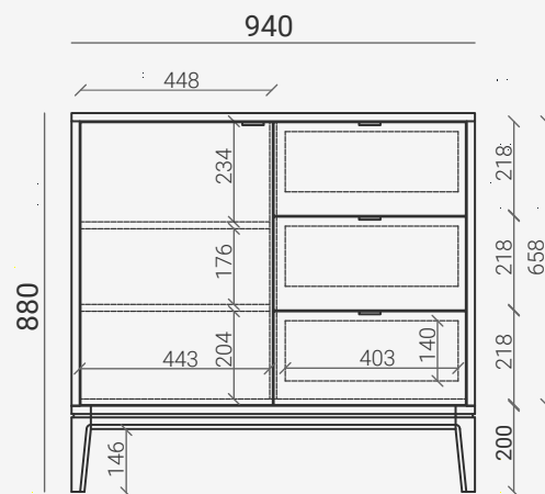
TL029 Д940 Ш400 В880
