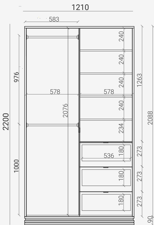
TLD218 Д1210 Ш600 В2200
