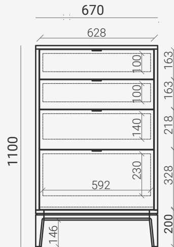
TL020 Д670 Ш450 В1100
