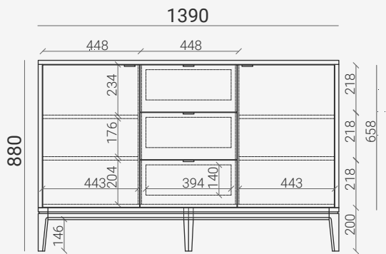
TL048 Д1390 Ш400 В880
