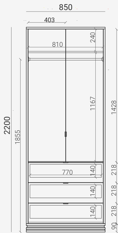
TLD208 Д850 Ш600 В2200
